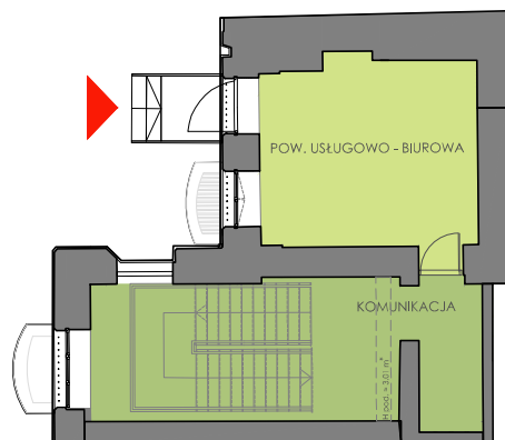
POZIOM 1
